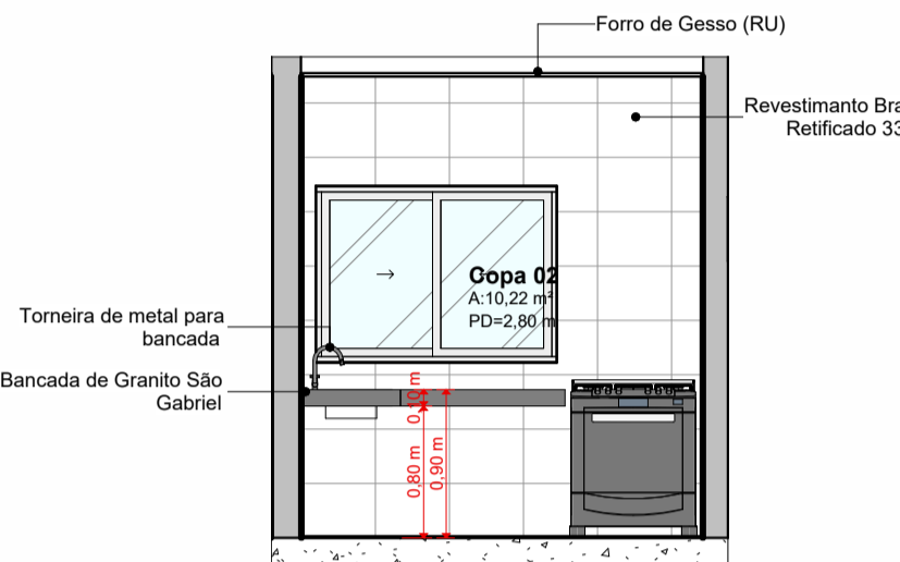
L2 Esc.: 1:50
