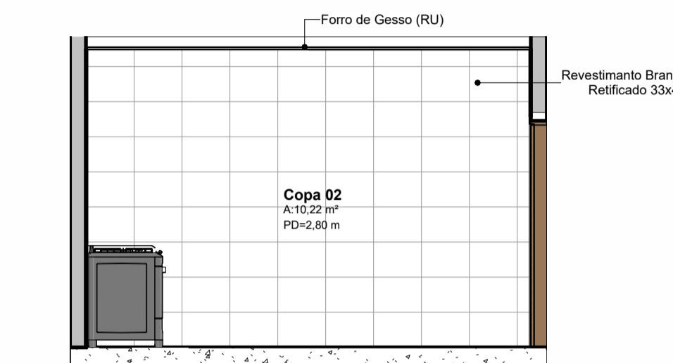
L3 Esc.: 1:50
