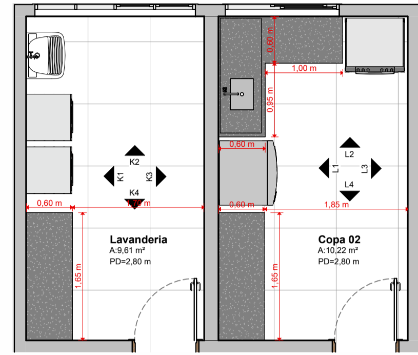
Lavanderia e Copa 02 Esc.: 1:50
