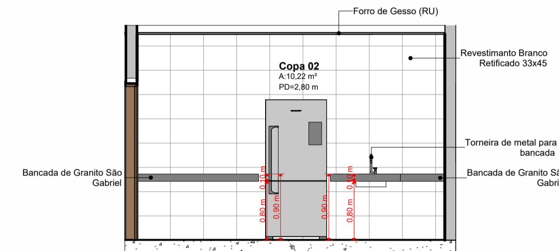
L1 Esc.: 1:50
