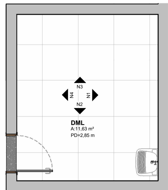
DML Esc.: 1:50
