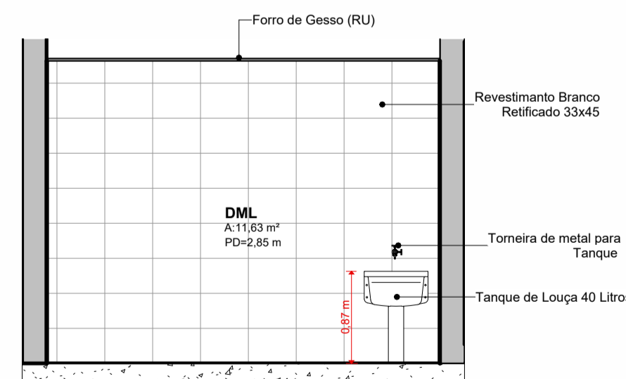
N1 Esc.: 1:50
