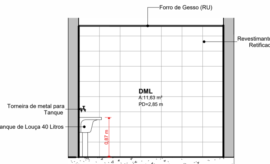
N2 Esc.: 1:50
