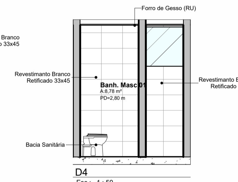
D4 Esc.: 1:50
