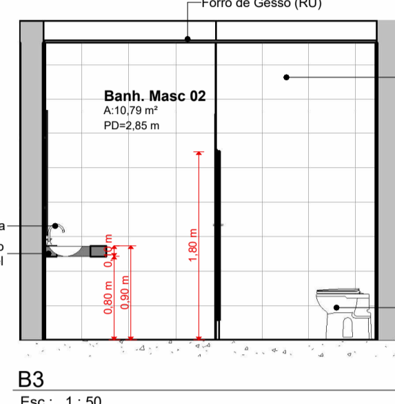
B3 Esc.: 1:50
