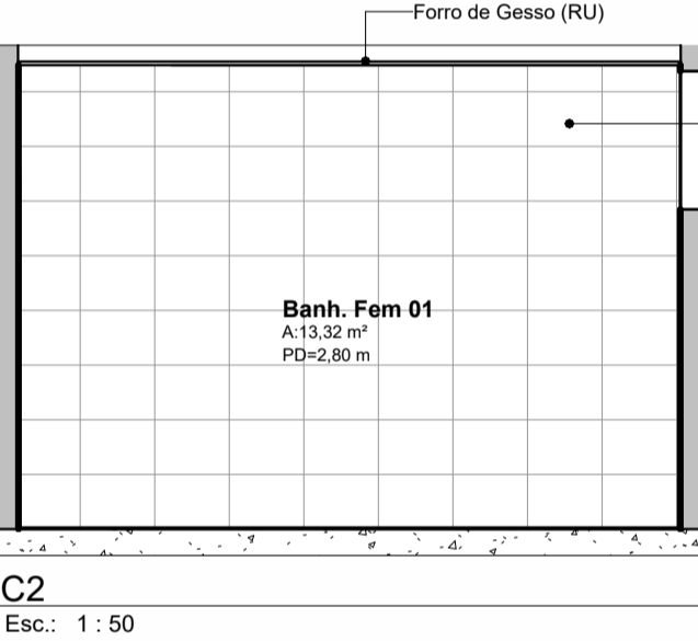
C2 Esc.: 1:50
