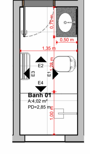
Planta Banheiro 01 Esc.: 1:50
