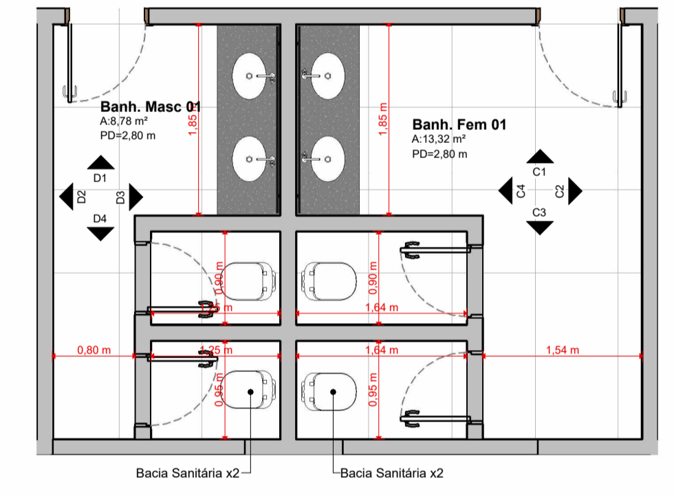
Planta Banh. Fem 02 e Masc 02 Esc.: 1:50
