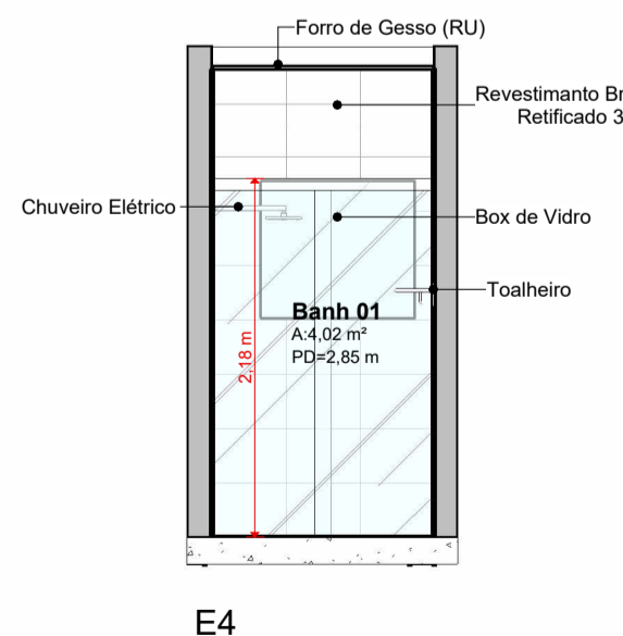
E4 Esc.: 1:50
