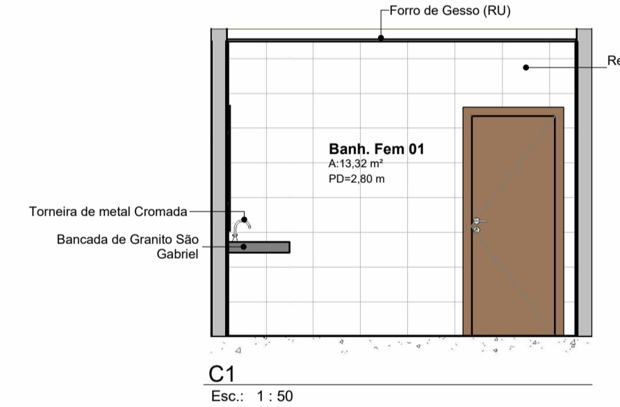
C1 Esc.: 1:50
