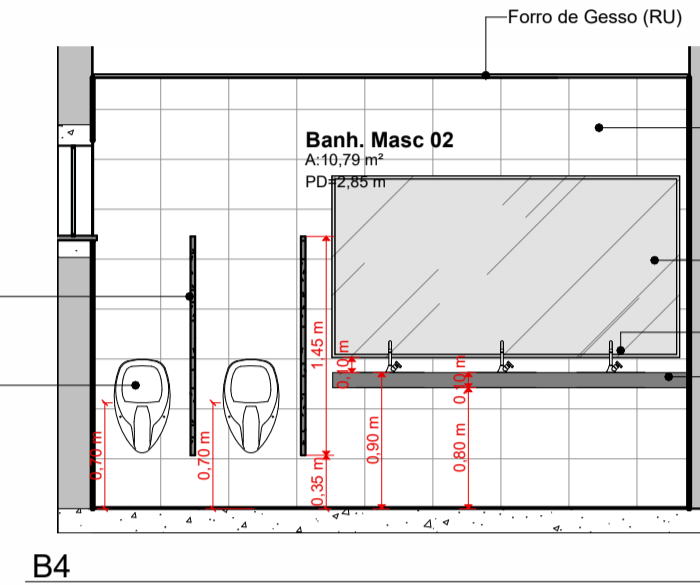
B4 Esc.: 1:50
