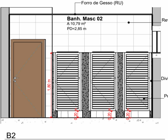
B2 Esc.: 1:50
