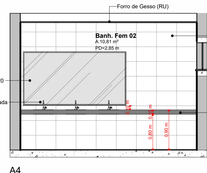
A4 Esc.: 1:50
