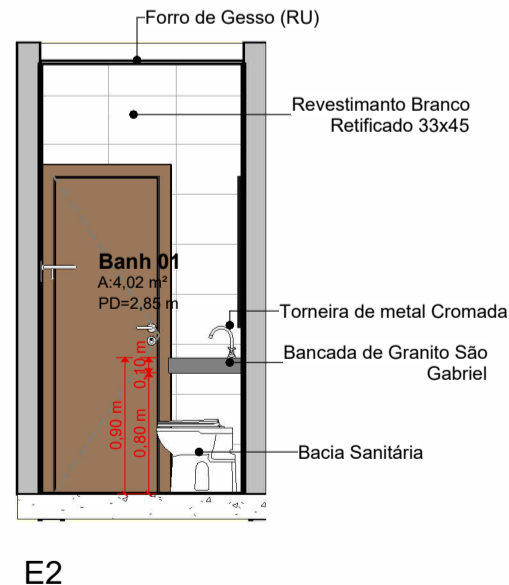
E2 Esc.: 1:50
