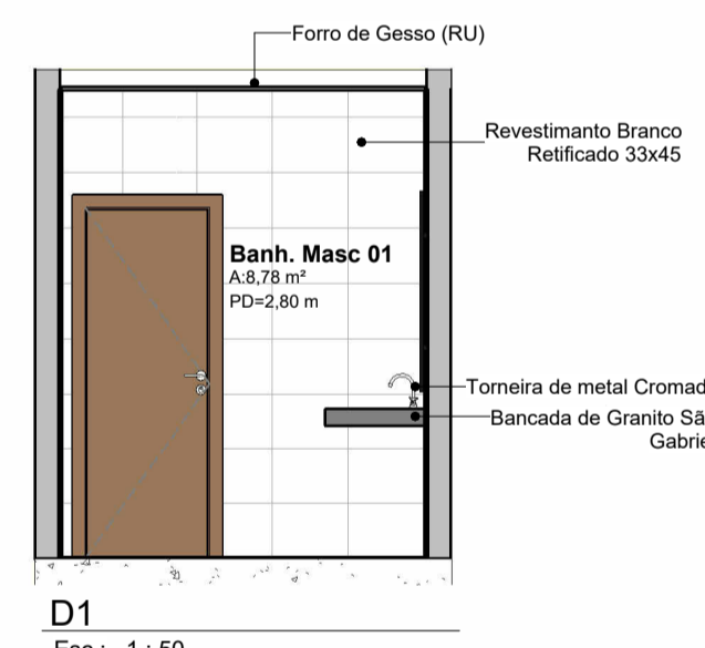
D1 Esc.: 1:50
