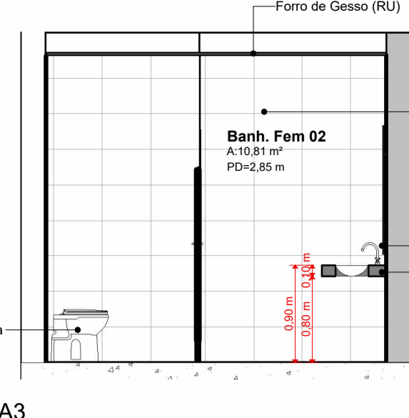
A3 Esc.: 1:50
