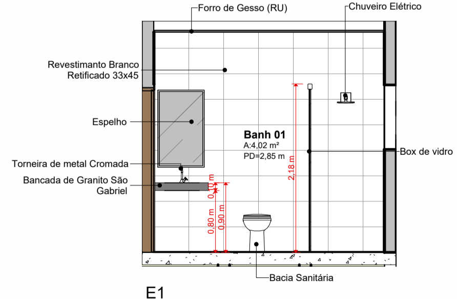
E1 Esc.: 1:50
