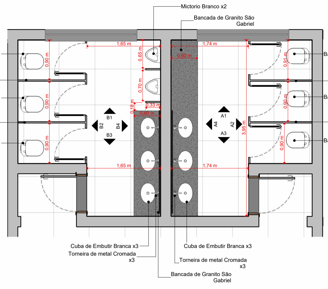
Planta Banh. Fem 02 e Masc 02 Esc.: 1:50
