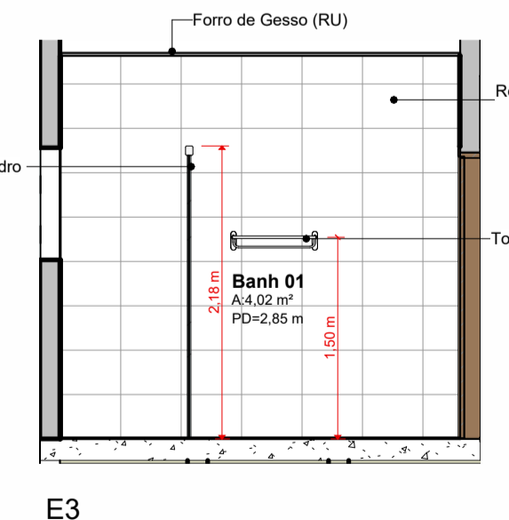
E3 Esc.: 1:50
