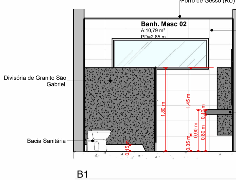
B1 Esc.: 1:50
