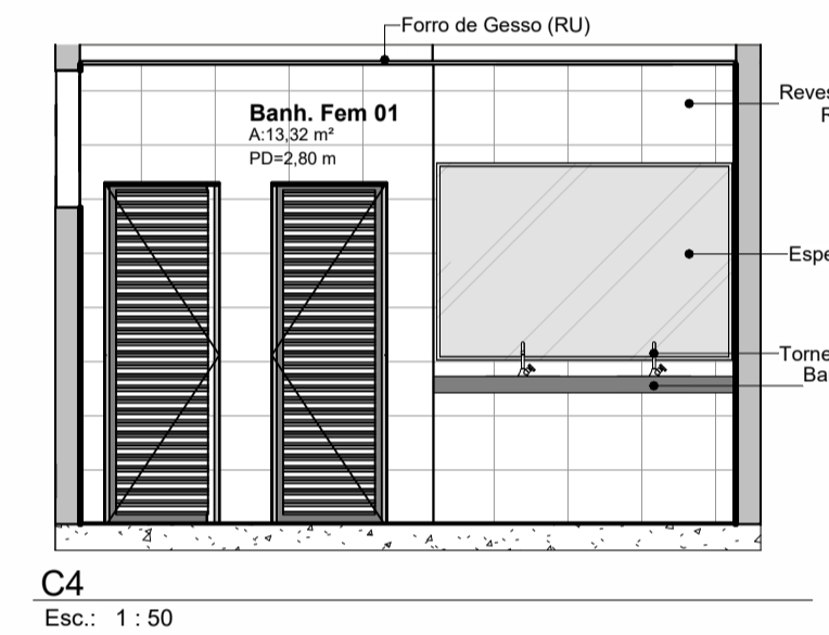
C4 Esc.: 1:50
