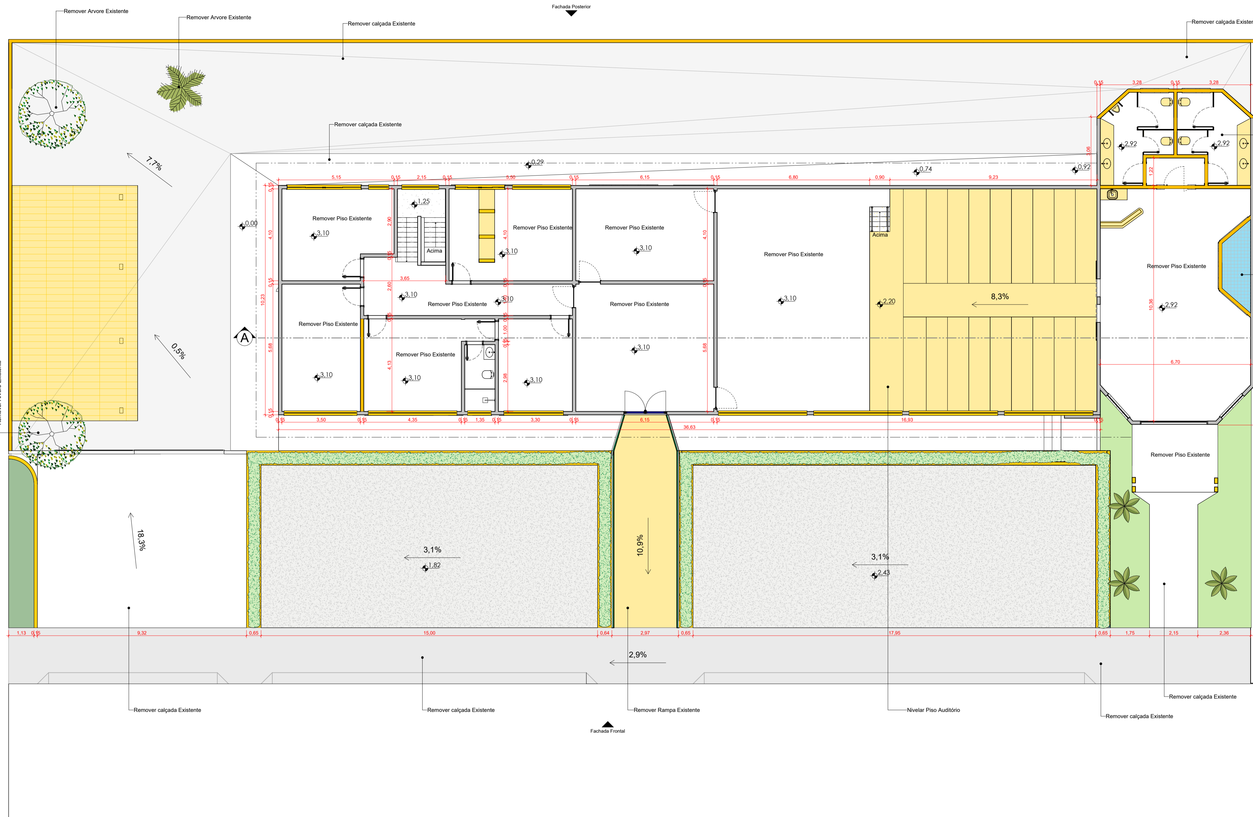
Planta 1º Pavimento à Demolir Esc.: 1:100
