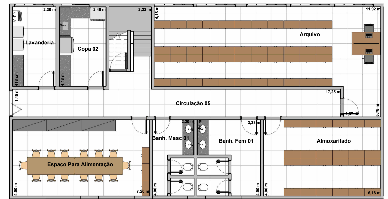
Planta de Layout Térreo Esc.: 1:100
