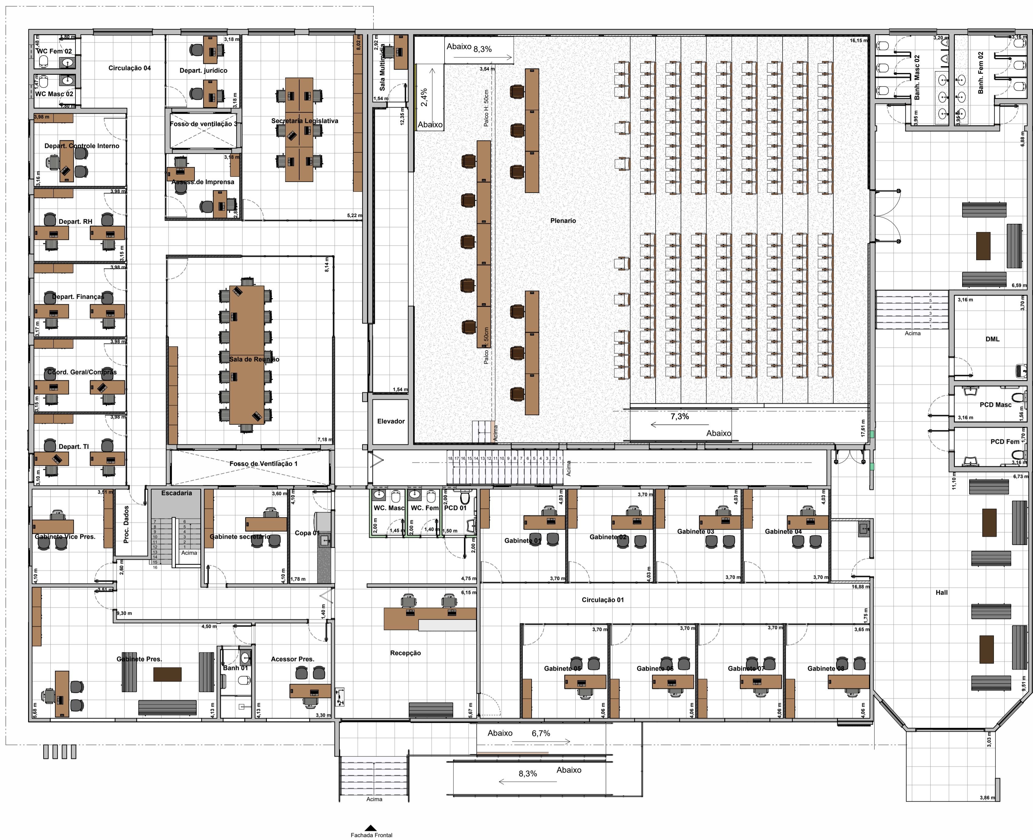
Planta de layout 1º Pavimento Esc.: 1:100
